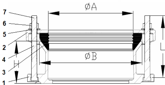
Рис.3. Муфта/адаптер ПФК
