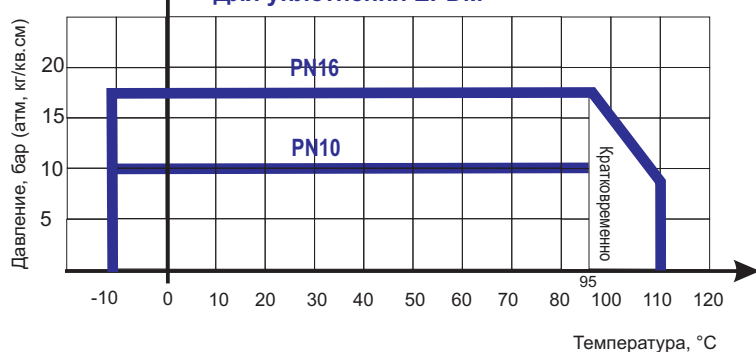
Диаграмма Давление / Температура для затвора поворотного дискового ABRA-BUV-FL226/263/266Dxxx DN 50-1000, PN 10 и PN 16
