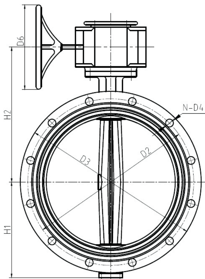
Чертеж габаритный затвора поворотного дискового чугунного фланцевого ABRA-BUV-FL226/263/266Dxxx с рукояткой (Н), редуктором (G) и голым штоком
