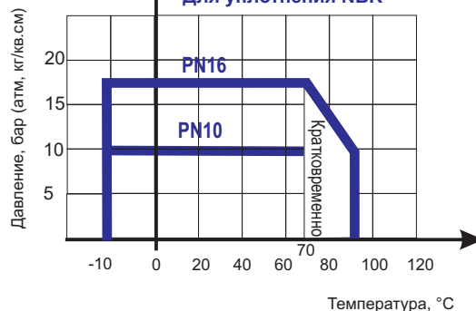
Диаграмма Давление / Температура для затвора поворотного дискового ABRA-BUV-FL226/263/266Dxxx DN 50-1000, PN 10 и PN 16
