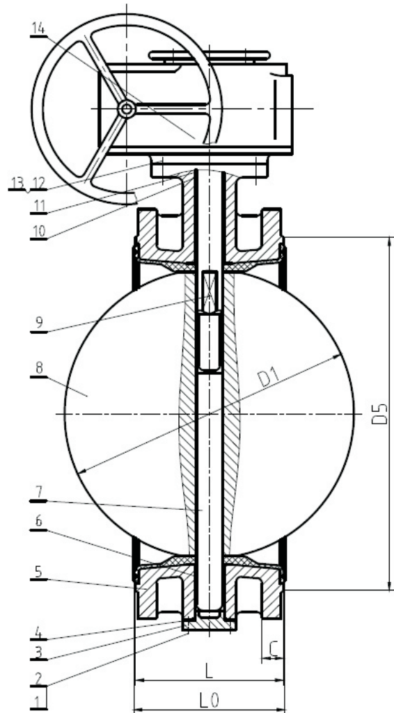
Чертеж габаритный затвора поворотного дискового чугунного фланцевого ABRA-BUV-FL226/263/266Dxxx с рукояткой (Н), редуктором (G) и голым штоком
