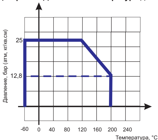
Диаграмма Давление / Температура для обратного клапана тарельчатого межфланцевого ABRA-D71
