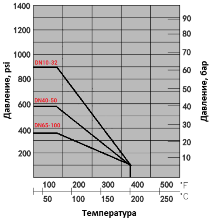
Рисунок 1 – Диаграмма «Температура-давление»
